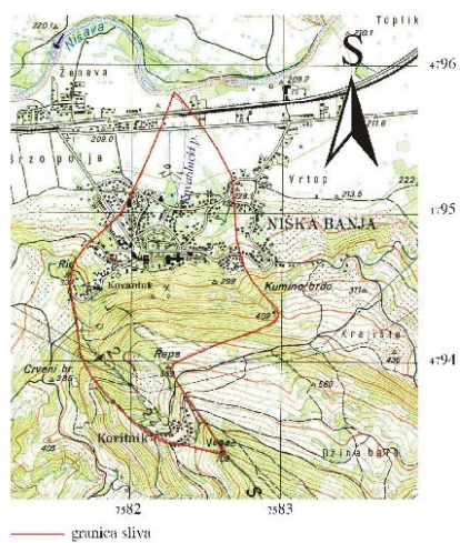
SITUACIJA SLIVNOG PODRUČJA KOVANLUČKOG POTOKA R = 1 : 25 000
